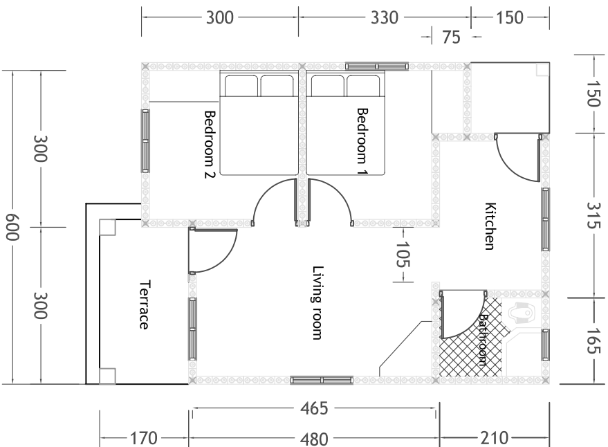
DENAH Skala 1 : 100
