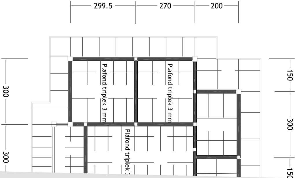
RENCANA Skala 1 : 10
